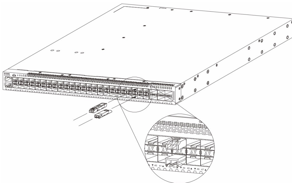
Рис. 12. Установка трансиверов SFP/SFP+ в порты SFP+
