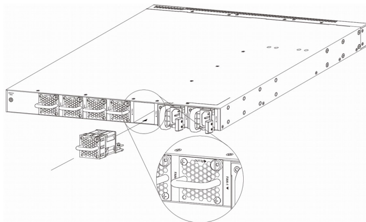
Рис. 18. Установка модуля вентилятора
