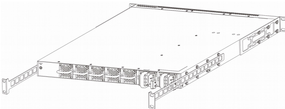
Рис. 9. Размещение кронштейнов для монтажа в стойку
