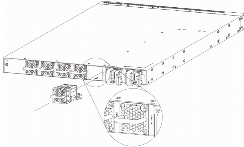
Figure 18. Installing a Fan Module
