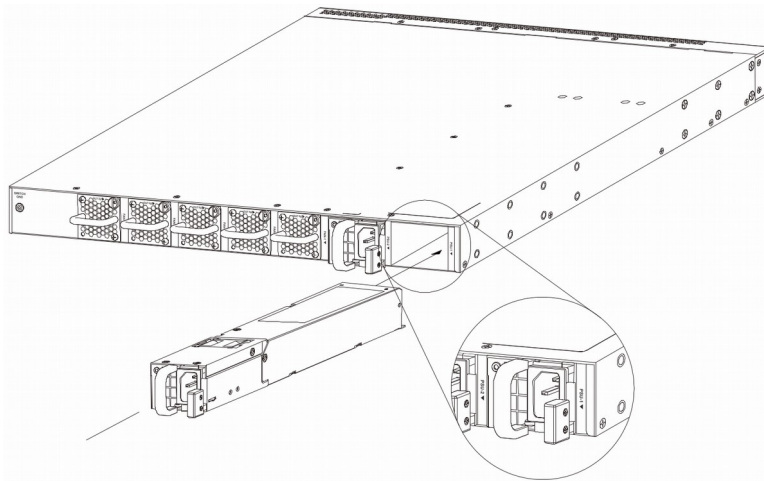
Рис. 13. Установка модуля питания переменного тока (AC)
