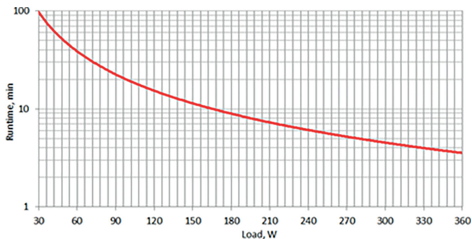
Figura 4. Grafico della durata della batteria di INFOPDU600 / INFOPDU600PL / INFOPDU600LCD
