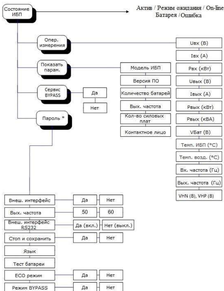
Рисунок 3 – Блок-схема ПО ИБП
