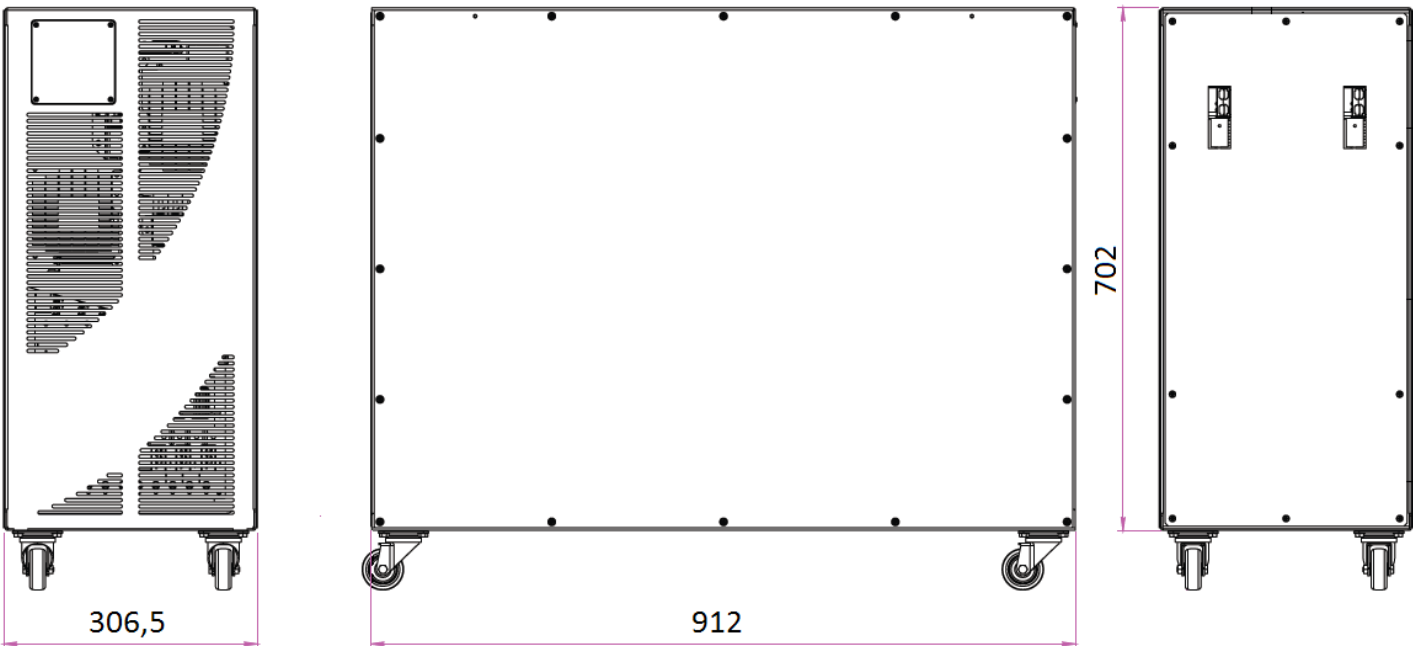
Рисунок 6. Внешний вид батарейного блока серии Solo MMB
