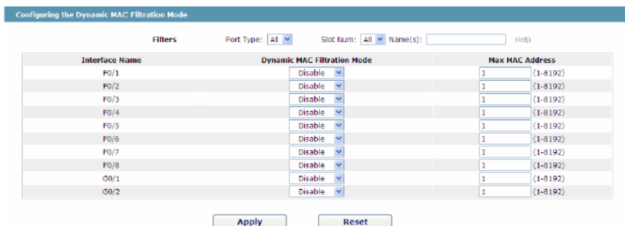
Рисунок 14 Настройки режима динамической MAC фильтрации
