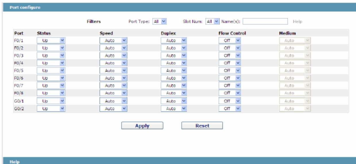
Рисунок 3 Настройка свойств портов
