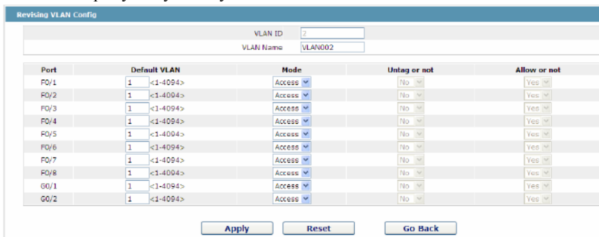
Рисунок 3 Изменение VLAN конфигурации
