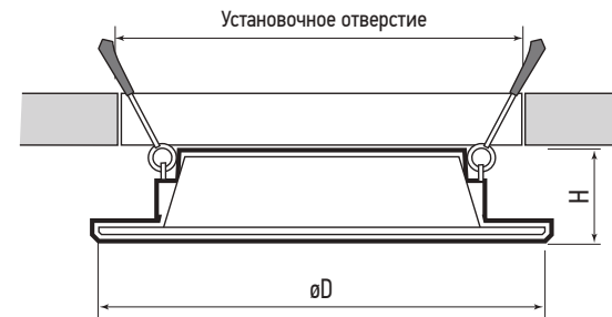
Рис. №1 Светильник PLED DL6
